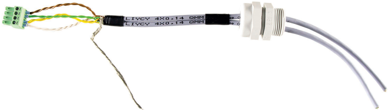
Fig.: Cablaggio campione al connettore a 4 poli della morsettiere
