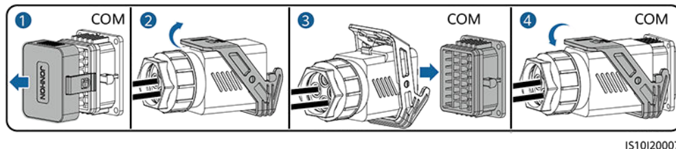
Figura 5-28 Fissaggio del connettore del cavo di segnale
