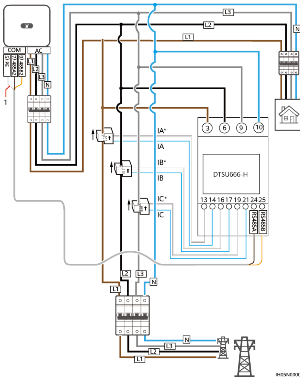
Figura 5-24 Collegamento dei cavi (Trifase a quattro fili)
