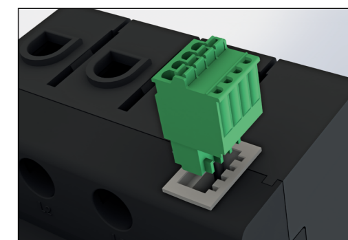
Figura: Energy Manager con connettore a spina su interfaccia RS485
