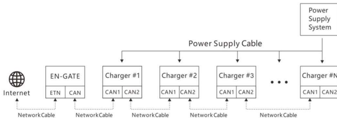
Figura 16 - Collegamento stazioni di ricarica
