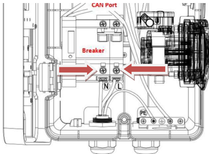
Figura 14 – Connessione dei cavi AC di uscita (2)
