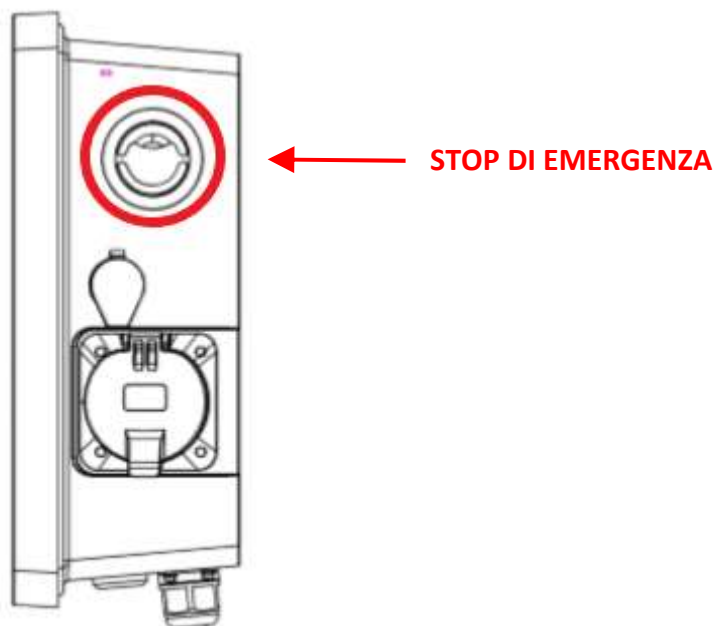
Figura 2 - posizionamento bottone di STOP
