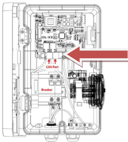
Figura 15 - Sistema di comunicazione
