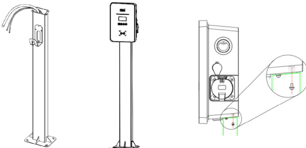
Figura 19 - Posizionamento pilone di supporto
