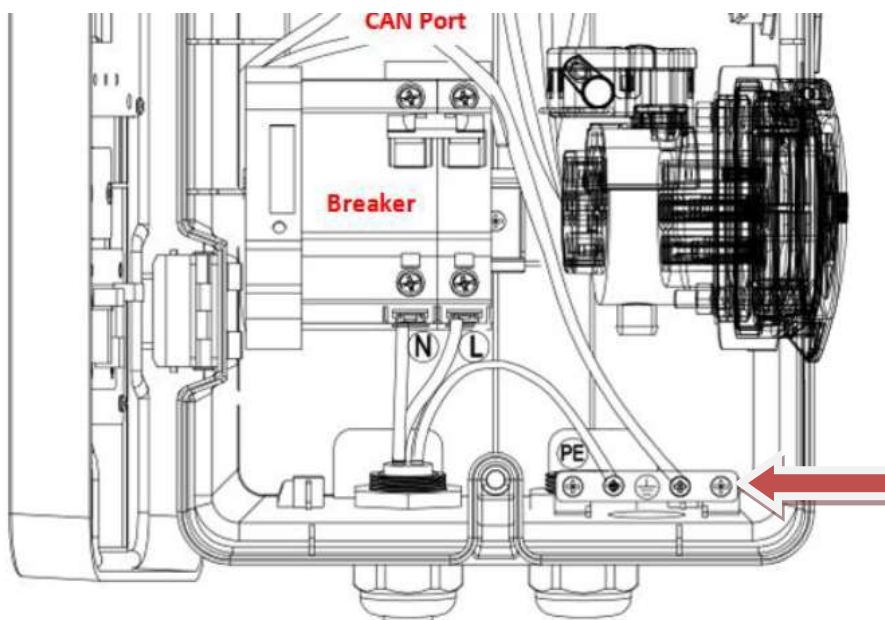
Figura 12 - Collegamento del terminale di terra
