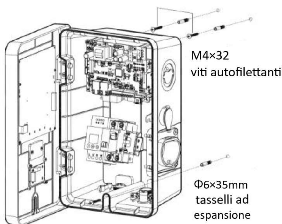
Figura 17 - Posizionamento viti per montaggio a parete
